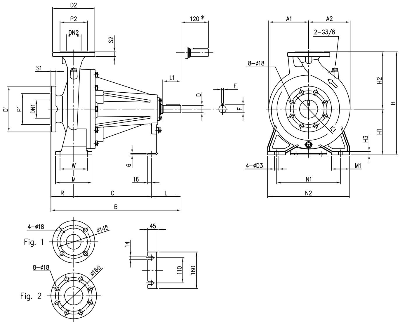
TABEAU DES DIMENSIONS
