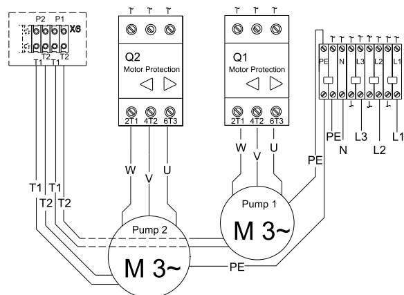
Fig. 30 Schéma de câblage, triphasé, Multilift MD/MLD.24.3.2, MD/MLD.32.3.2 et MD/MLD.38.3.2 avec disjoncteur
