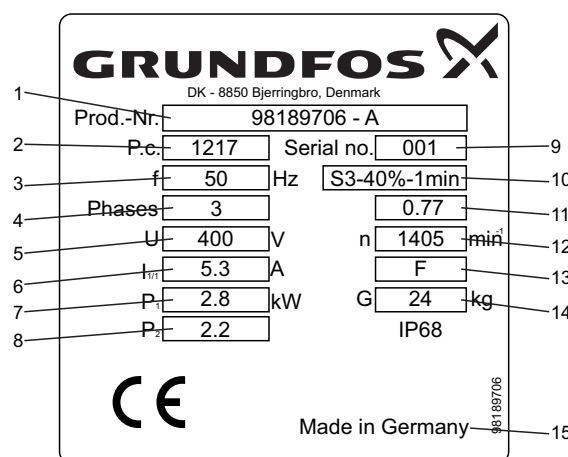
Fig. 4 Plaque signalétique du moteur
