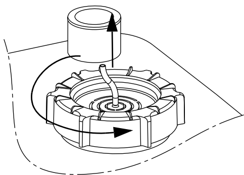
Fig. 35 Retrait du capteur de niveau
