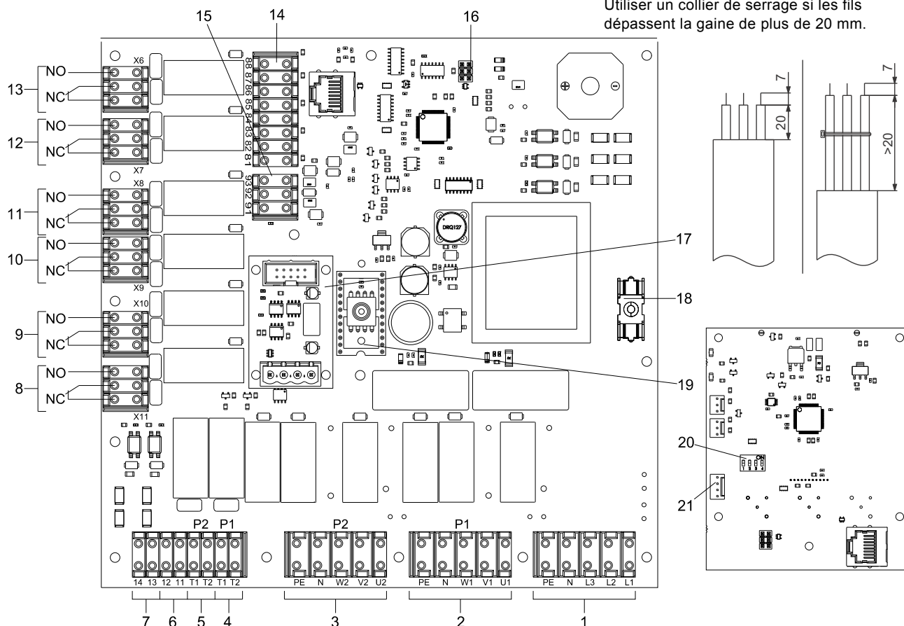
Fig. 10 Structure interne du LC 221 (circuit imprimé triphasé par exemple)
