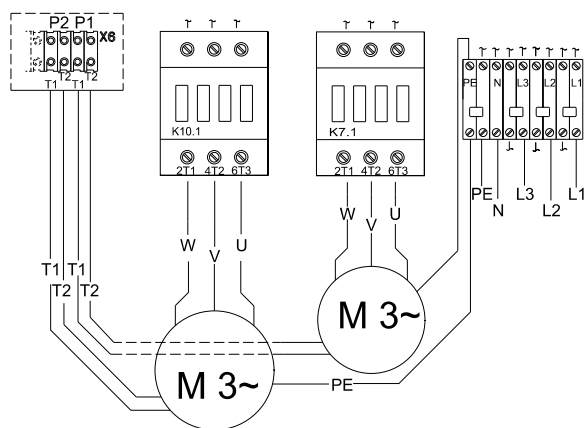
Fig. 29 Schéma de câblage, triphasé, Multilift MD/MLD.22.3.4 avec contacteurs
